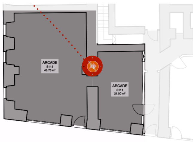
(Above) Artjugg Gallery Floor Plan 11, rue de l'Hôtel de Ville 1204 Genève
